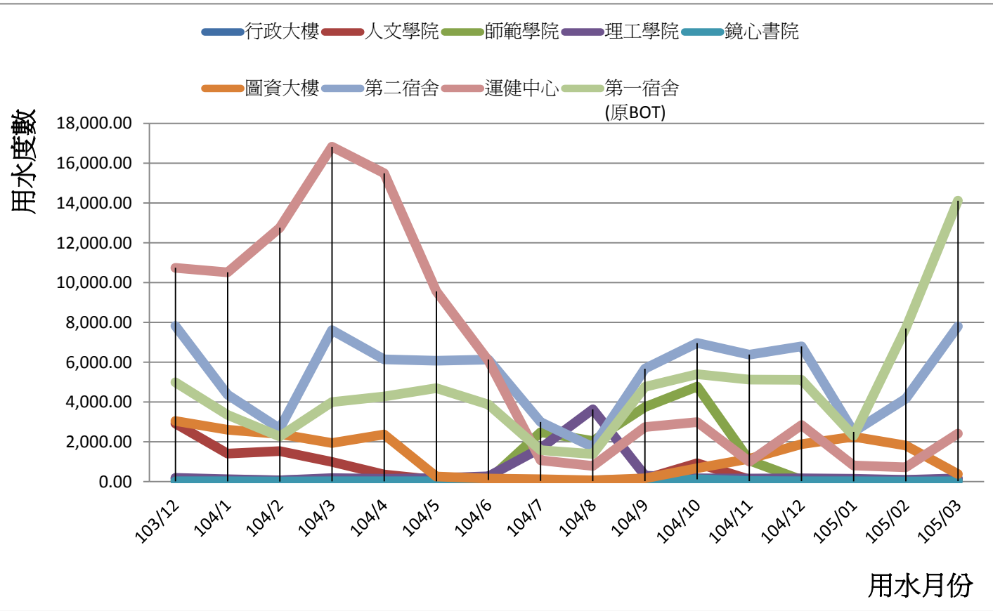
103年12月至105年3月校本部各建物單位樓板面積月用水量統計圖
