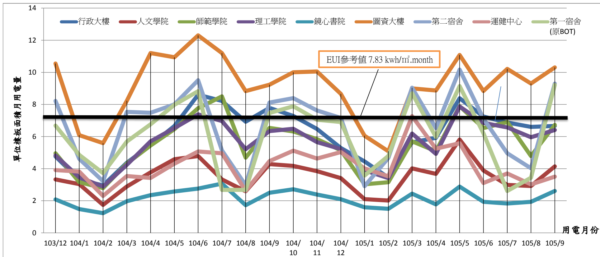
103年12月至105年9月各建物單位樓板面積月用電量
